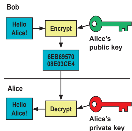
Εικόνα 6.1 Ασύμμετρη Κρυπτογράφηση
